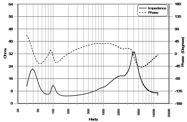
Impedance/Phase
