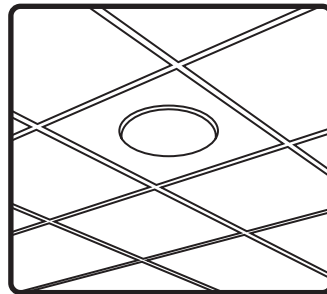
10. Done!
